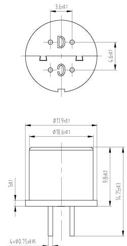
图 1： 传感器外形结构
