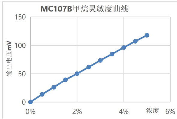
图 3：灵敏度曲线
